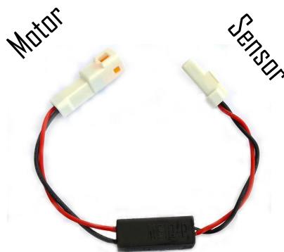
Abb. 6 Anschluss Motorseite / Geschwindigkeitssensorseite
