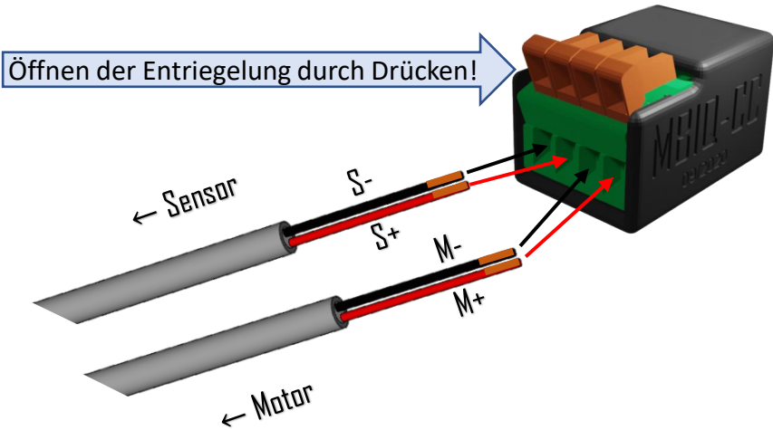
Abb. 4: Zuordnung der Sensorleitungen
