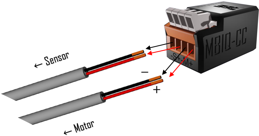
Abb. 4: Zuordnung der Sensorleitungen
