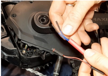
Abbildung 5: Schrumpfschlauch zur Sicherung der Verbindung
