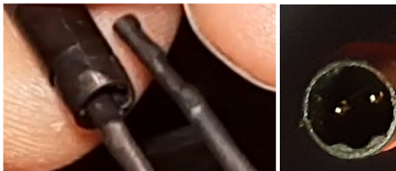
Abbildung 6: MBEvo mit Sensor verbinden
