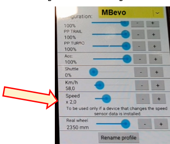
Abbildung 14: BLEvo und Teilung durch 2, Tuning aktiviert
