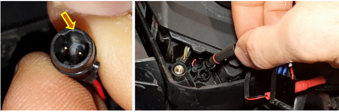
Abbildung 8: MBevo Verbindung im Motorraum herstellen
