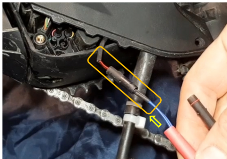
Abbildung 7: Schrumpfschlauch über die Verbindung
