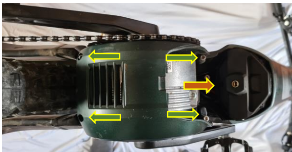
Abbildung 2: Motorabdeckung / Akku entfernen
