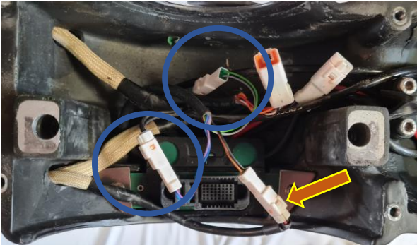
Abbildung 5: Lichtanschluss
