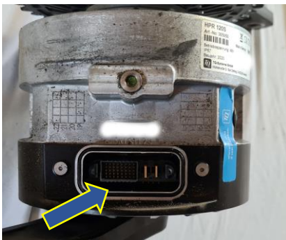
Abbildung 7: Gummidichtung überprüfen
