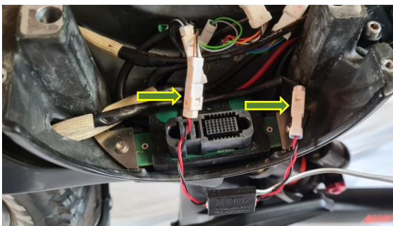
Abbildung 6: Modul installieren
