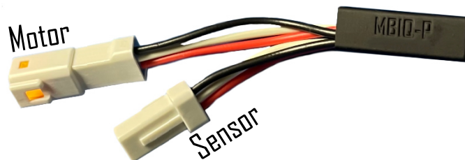
Abbildung 3: Tuning-Modul verbinden
