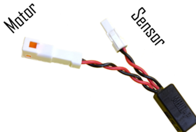
Abbildung 3: Tuning-Modul verbinden
