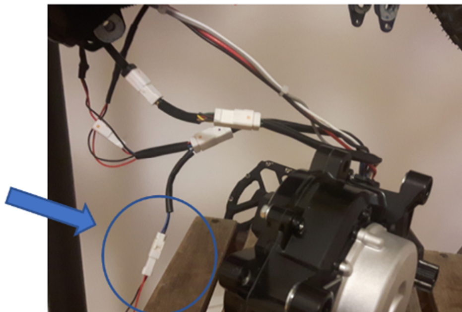
Abbildung 2: Steckerposition des Geschwindigkeitssensors
