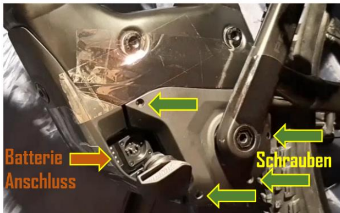
Abbildung 1: Batterieanschluss und Gehäuseabdeckung
