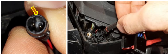
Abbildung 5: MBIQ-P Verbindung im Motorraum herstellen
