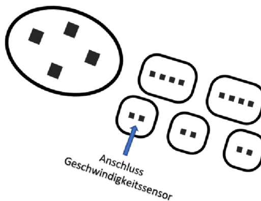
Abbildung 2: Steckerposition des Geschwindigkeitssensors
